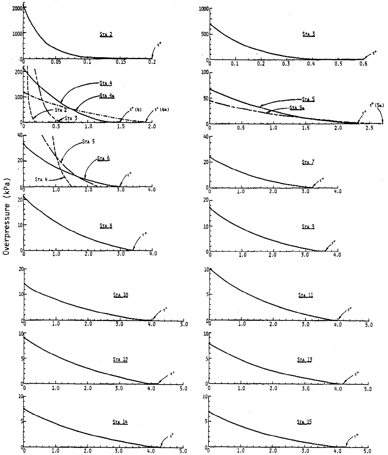
Fig. 17. Flat Terrain Overpressure Pulses of Sta 2 Through Sta 15.
