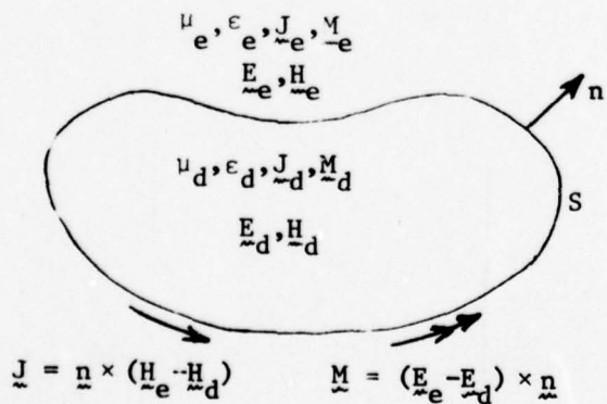
Fig. A-3. Composite Situation.
