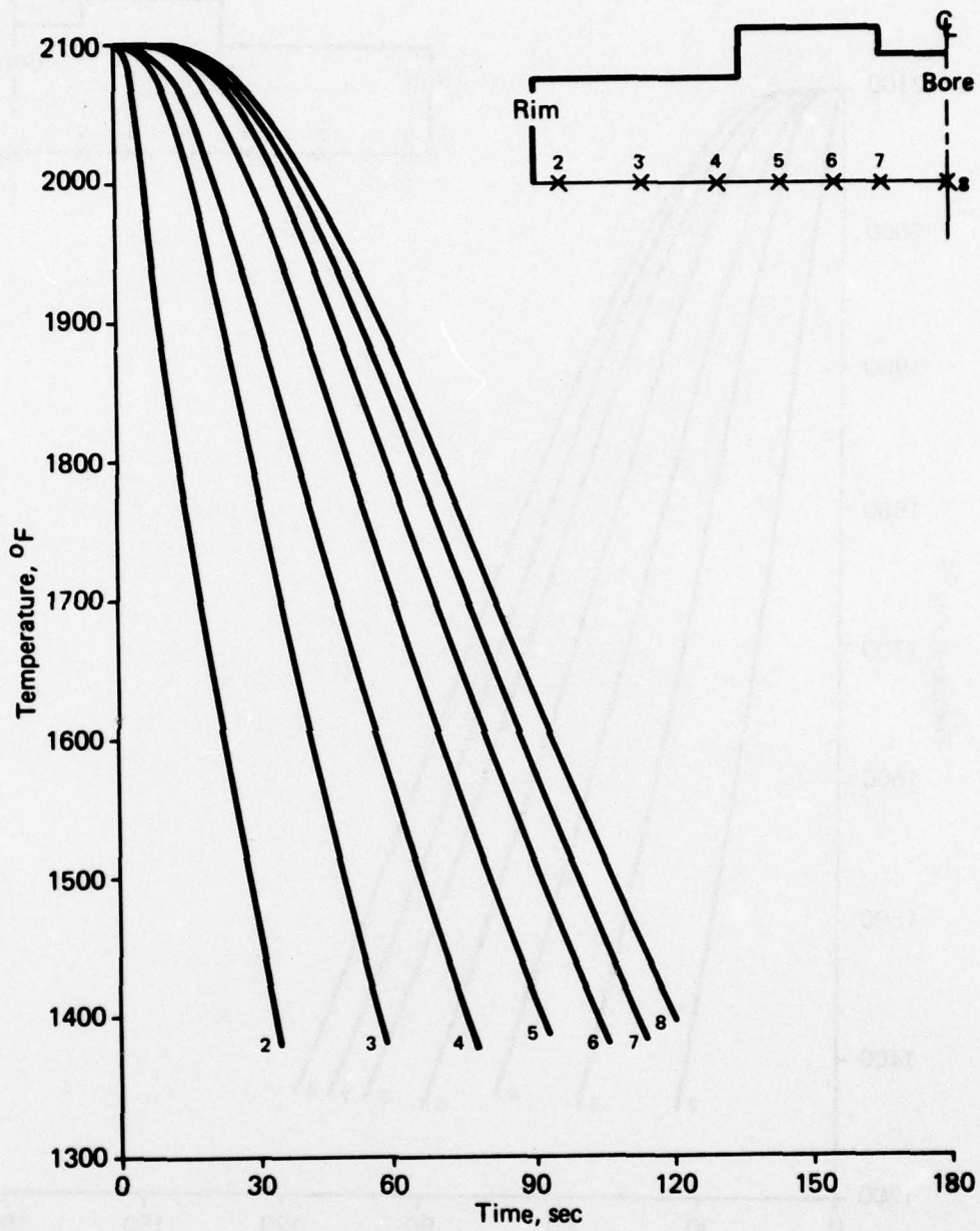
(d) 400°F salt quench
