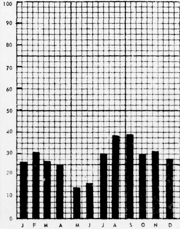
SUPERREFRACTIVE
