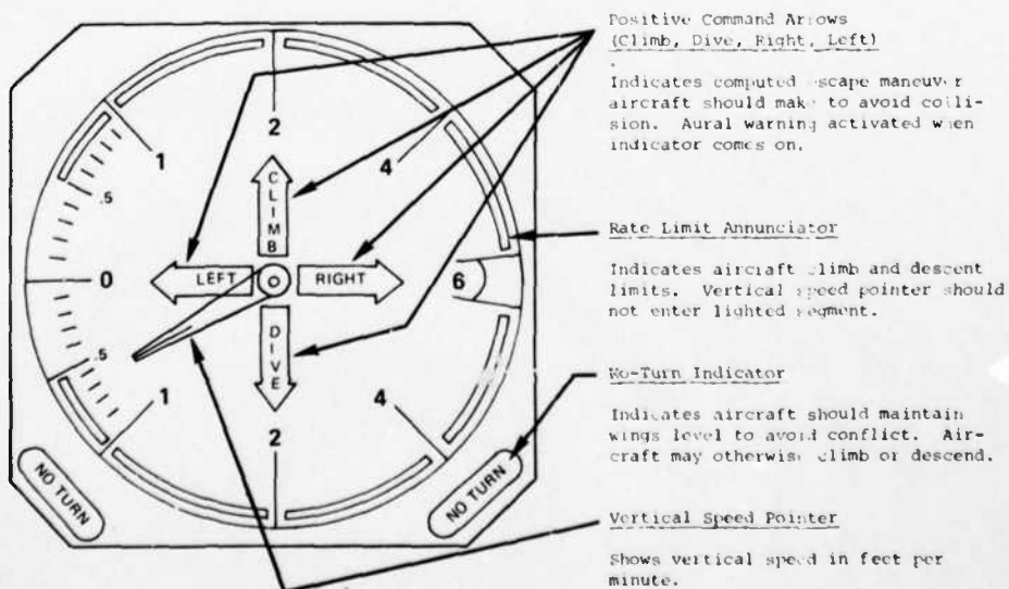
IVSI Indicator
