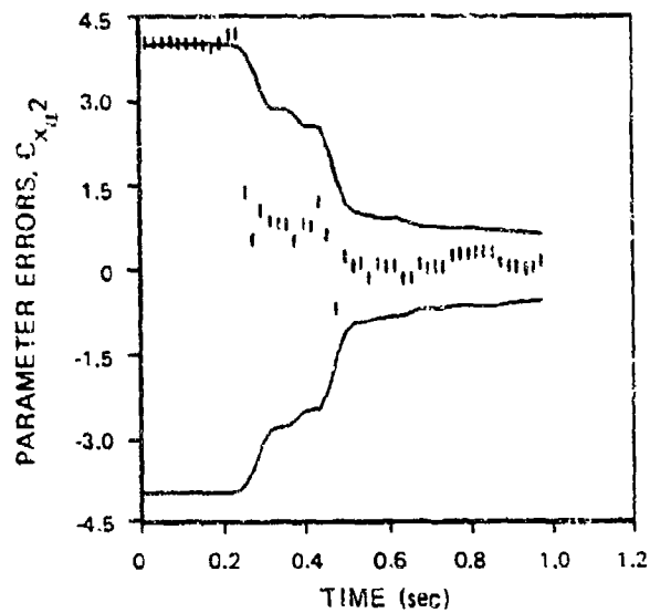
(b) PARAMETER ERRORS, C_{x_{d^2}}
