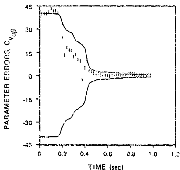
(l) PARAMETER ERRORS, C_{Y\beta a\delta}
