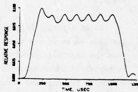
(d) B_t/B_r = 125 < N_c
