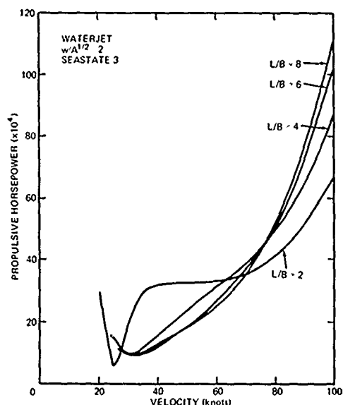
Fig. 23c - 10,000 Ton SES
