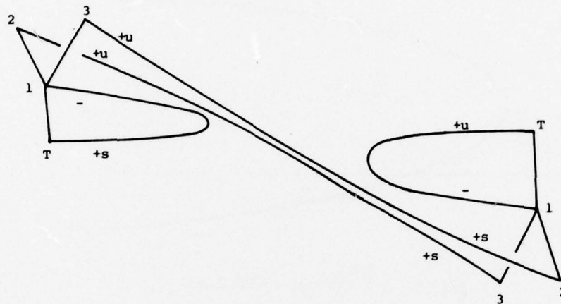
Figure 2.4e 1 : III 2 , \epsilon > 0 , k odd
