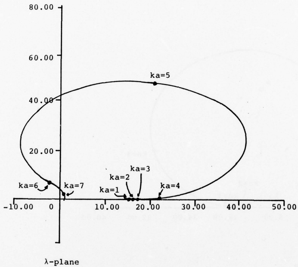
Figure 8. \lambda_n(ka) , n = 7
