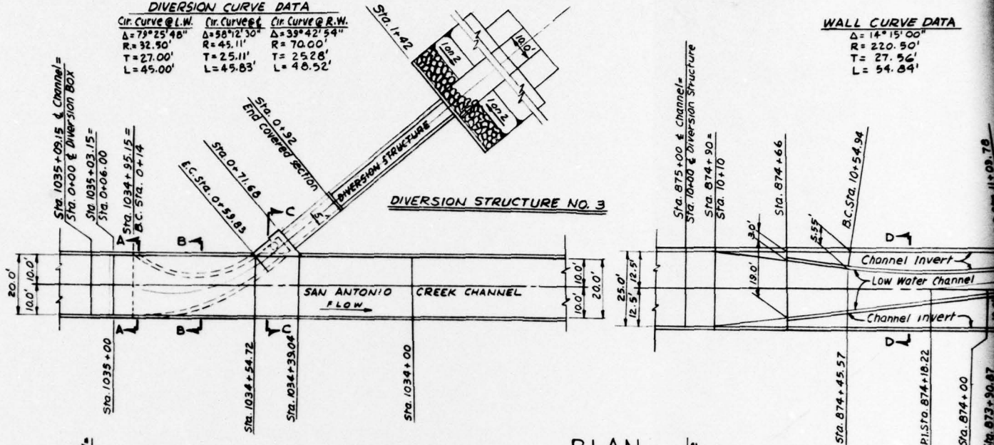
PLAN SCALE: 1" = 20'.
