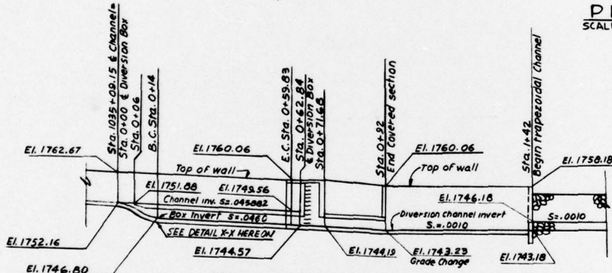
PROFILE - DIVERSION CHANNEL SCALE: 1" = 20'.
