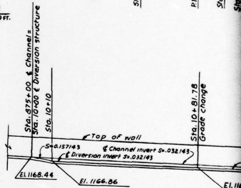
PROFILE - DIVERSION CHANNEL SCALE: 1" = 20'.
