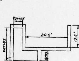
PROFILE - DIVERSION CHANNEL SCALE: 1" = 20'.
