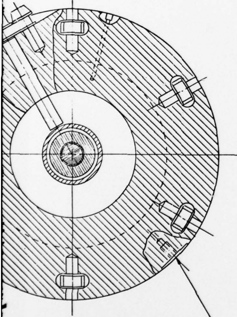
SECT D-D SCALE: 2 X 1
