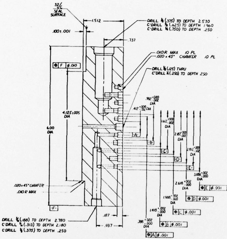
SECTION A-A
