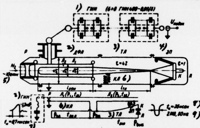
Fig. 1. Schematic diagram of the apparatus ESU. KEY: 1) GIN; 2) DFL; 3) TL; 4) EP; 5) 10 atm; 6) KL; 7) \mu\text{s} ; 8) ns; 9) kA.
