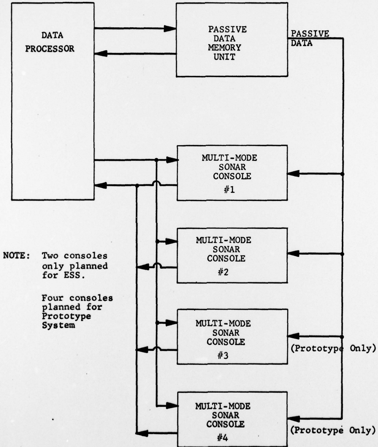
FIG. 2-1. DISPLAY SEGMENT
