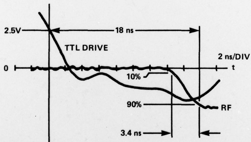
b) RF TURN-ON TRANSIENT
