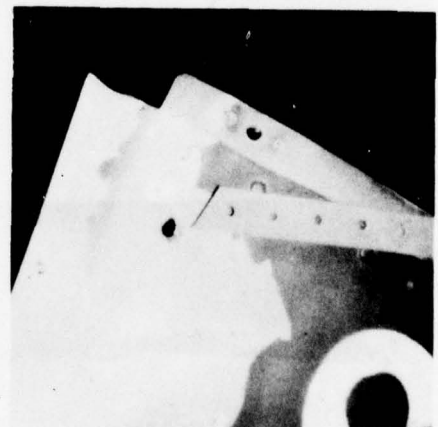
FIG. 6 : LIGHTNING STRIKE ON GAZELLE FIN
