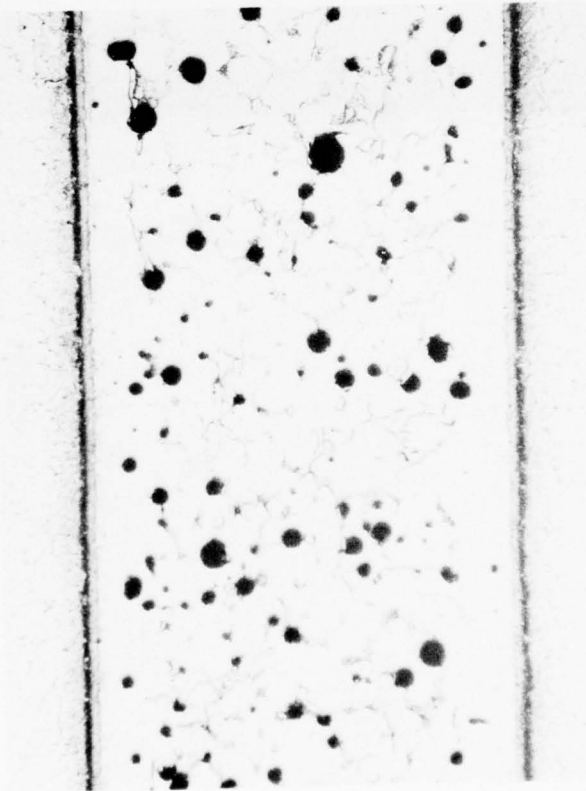
a. Kallings Etch 50X
