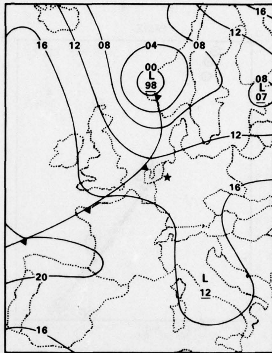
5 AUGUST 1977 0600 GMT
