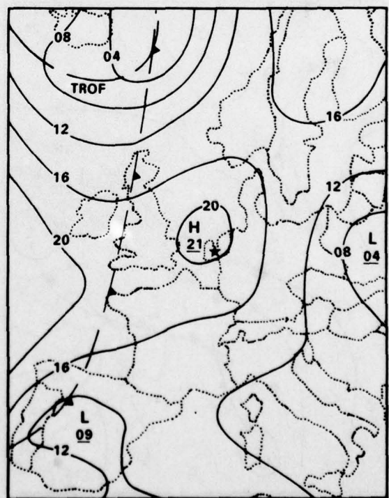
4 AUGUST 1977 0600 GMT
