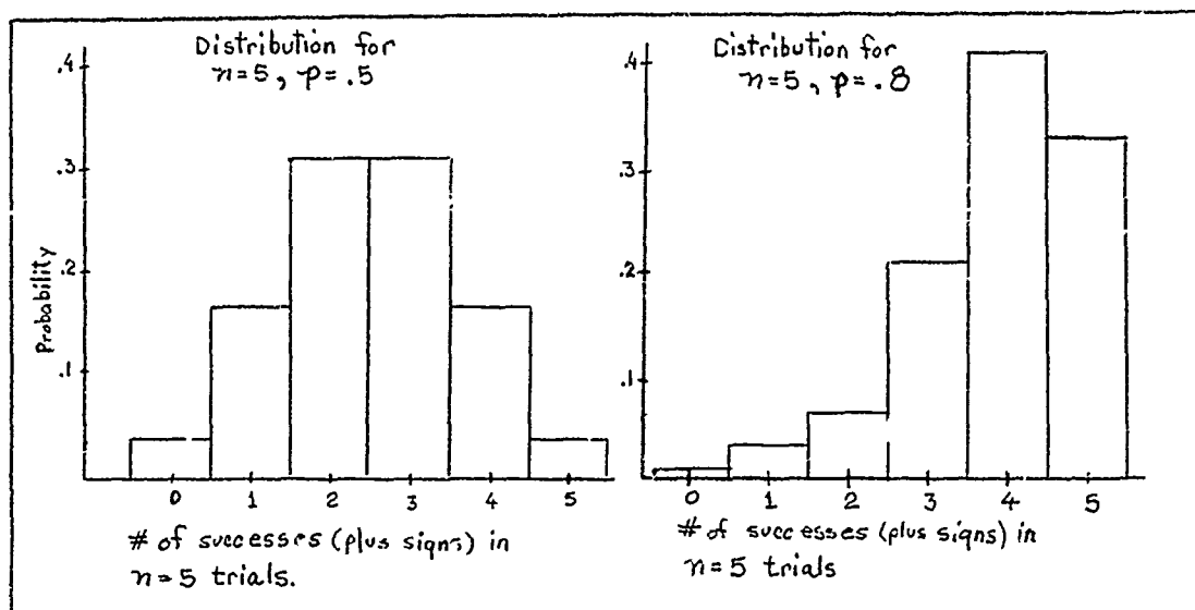
Fig 11. The Binomial Distribution
