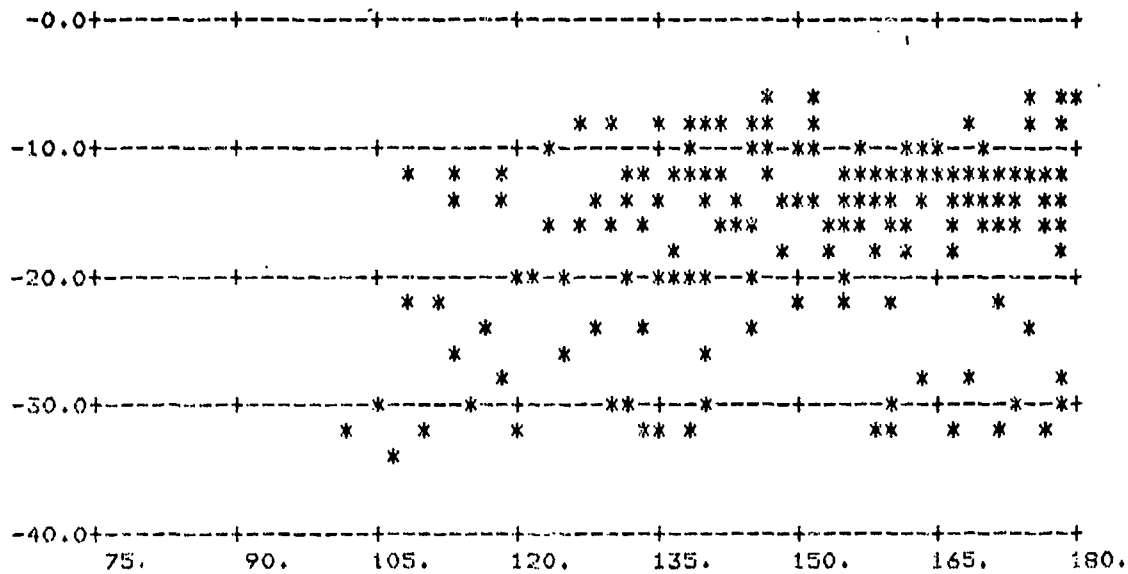
FIGURE A-26. \sigma_O vs \phi_S ; \theta_s = 80^\circ , \theta_i = 70^\circ
