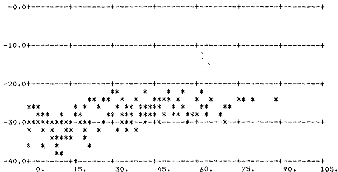
FIGURE A-27. \sigma_0 vs \phi_s ; \theta_s = 80^\circ , \theta_i = 70^\circ
