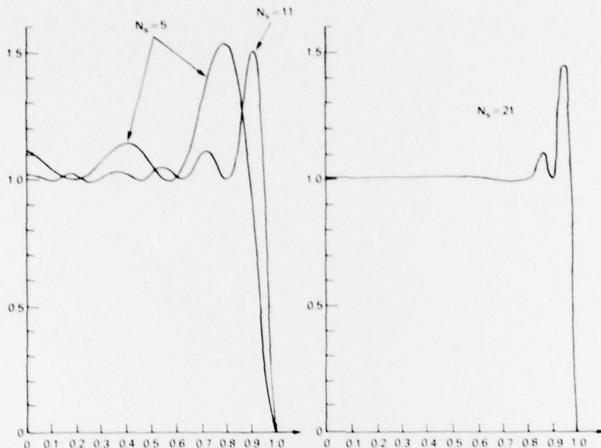
Fig. 2 - V_b/V_c vs \nu/W
