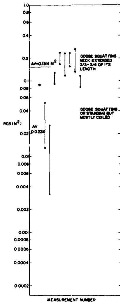
a. Horizontal Polarization
