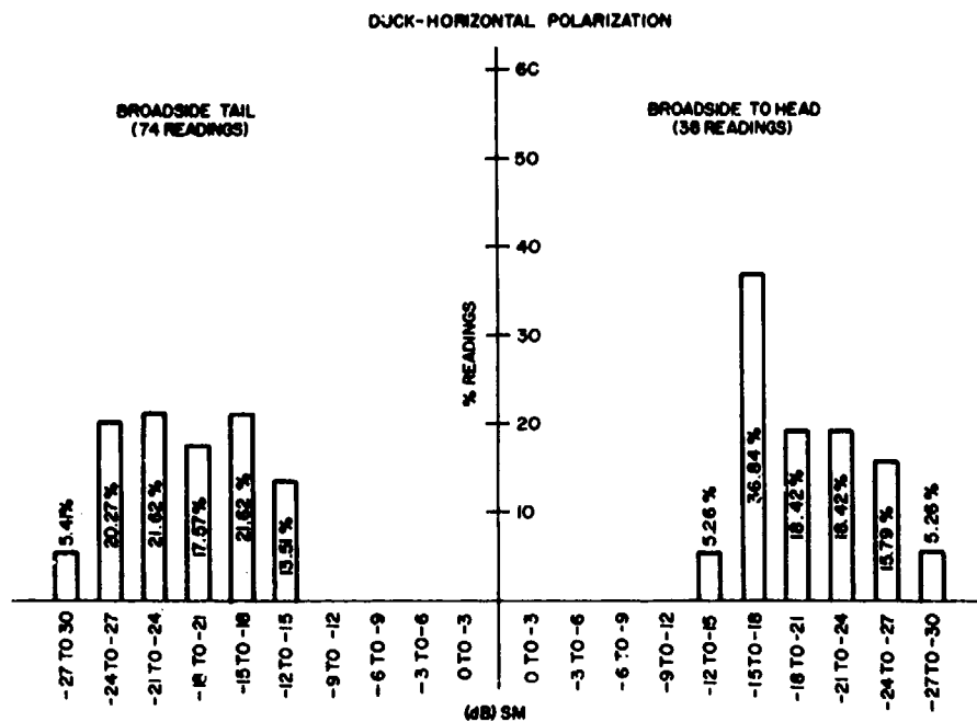
a. Duck Horizontal Polarization
