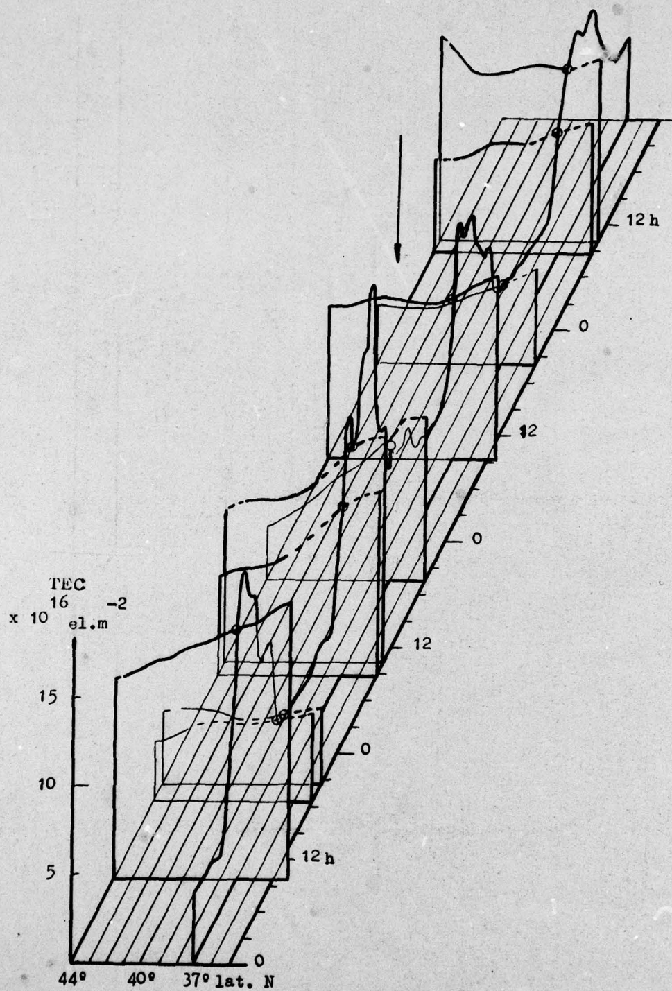
Fig. 4.- INTASAT - ATS/F data comparison
