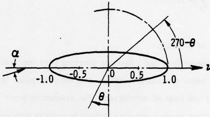
Fig. 7. Coordinate v
