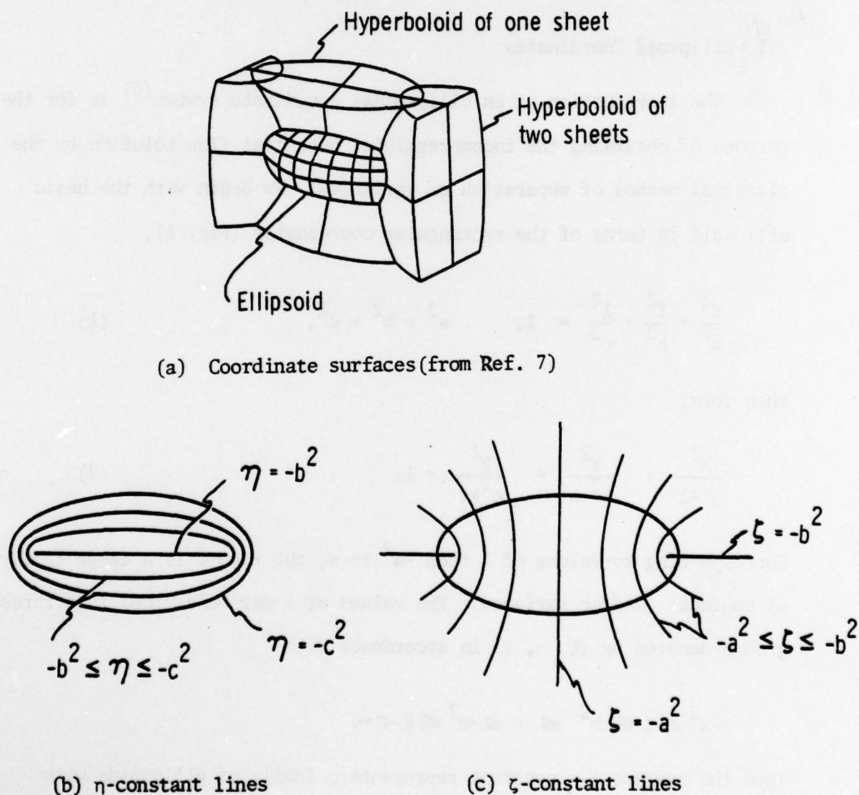
Fig. 2. Ellipsoidal coordinates
