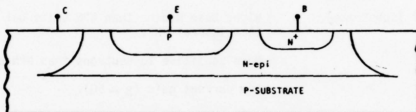
(b) Vertical (Substrate) PNP transistor.
