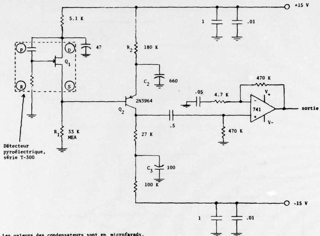
FIGURE 4 - Détecteur et préamplificateur
