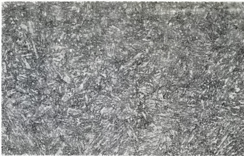
5(a) OD - Martensite - Bainite
