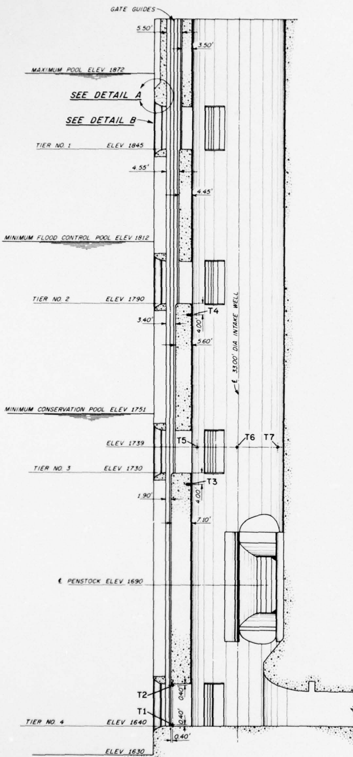
SECTION A-A
