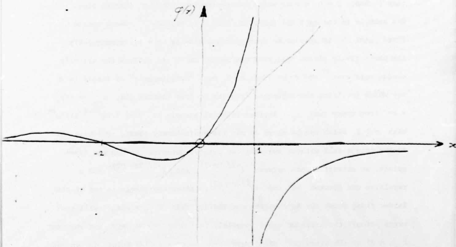
Fig 2 : q(x) = \frac{x(x+2)}{(1-x^2+2x+2)}
