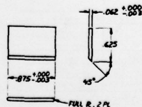
-015 BLADE
