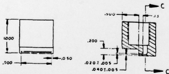
-019 NOZZLE TIP
