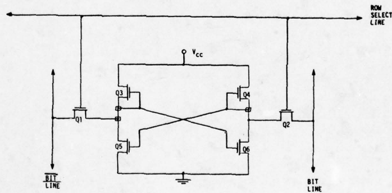
b) SCHEMATIC
