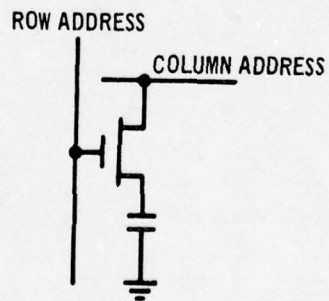
b) SCHEMATIC
