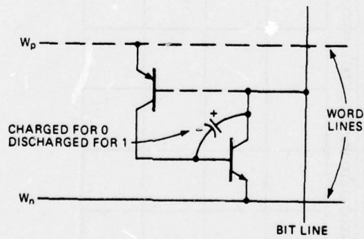
B) SCHEMATIC
