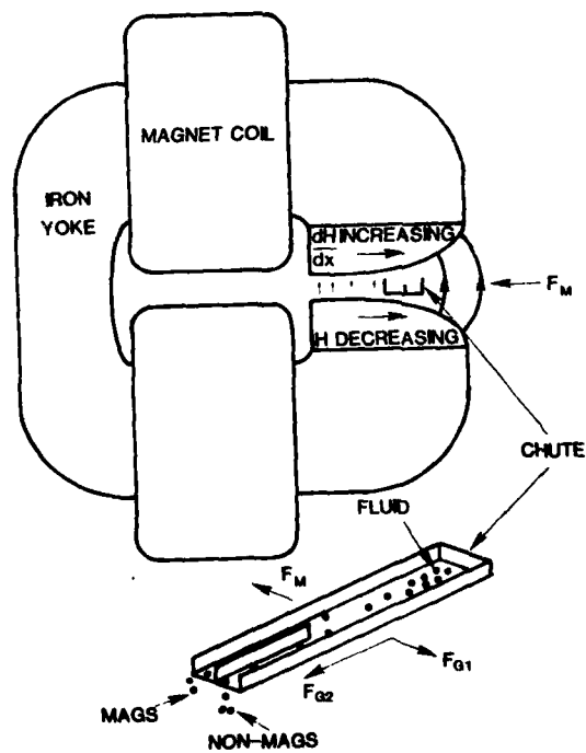
Fig. 7 Frantz-Isodynamic separator
