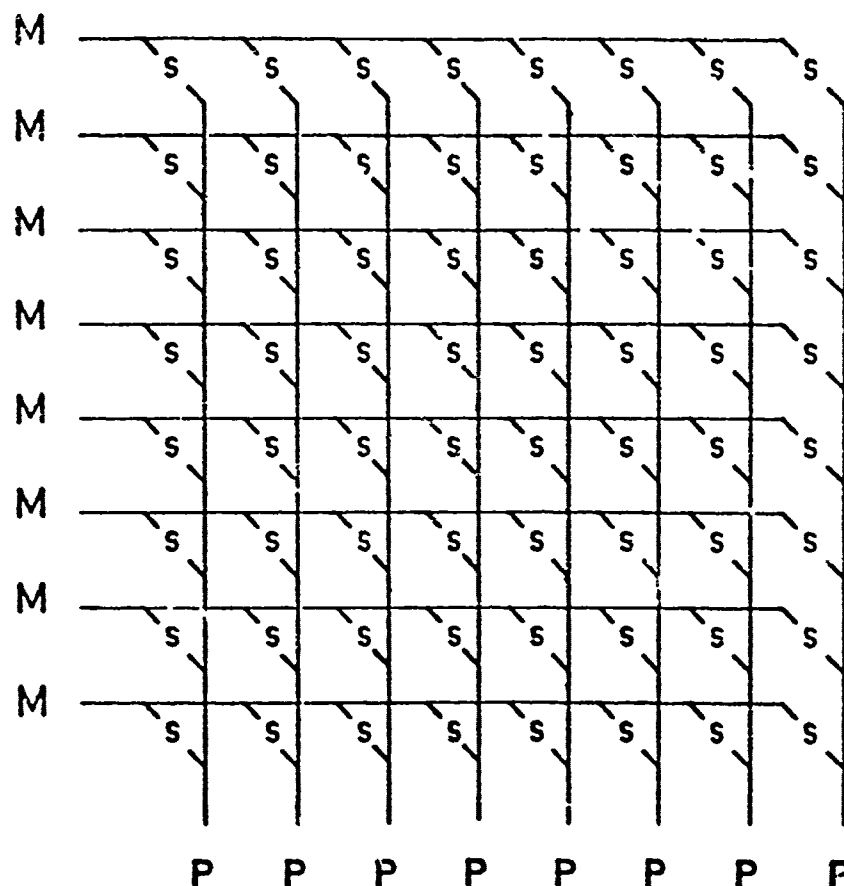
Fig. 3.2 Carnegie Mellon C.mmp
