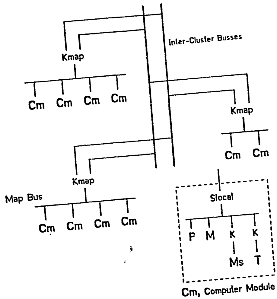
Fig. 3.4 Carnegie Mellon Cm*
