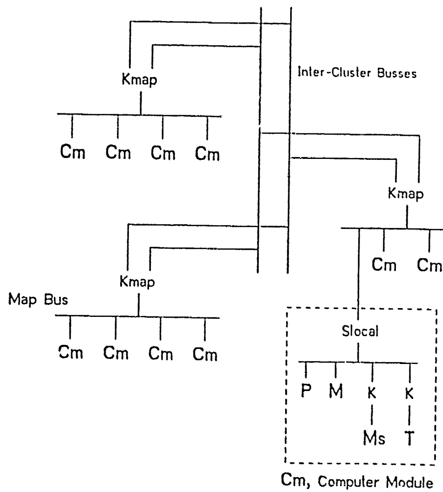
Fig. 6.2 Cm*
