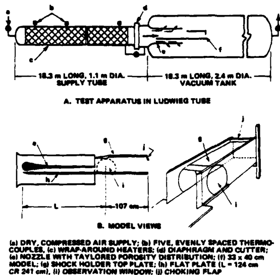
Fig. 2 Test apparatus.
