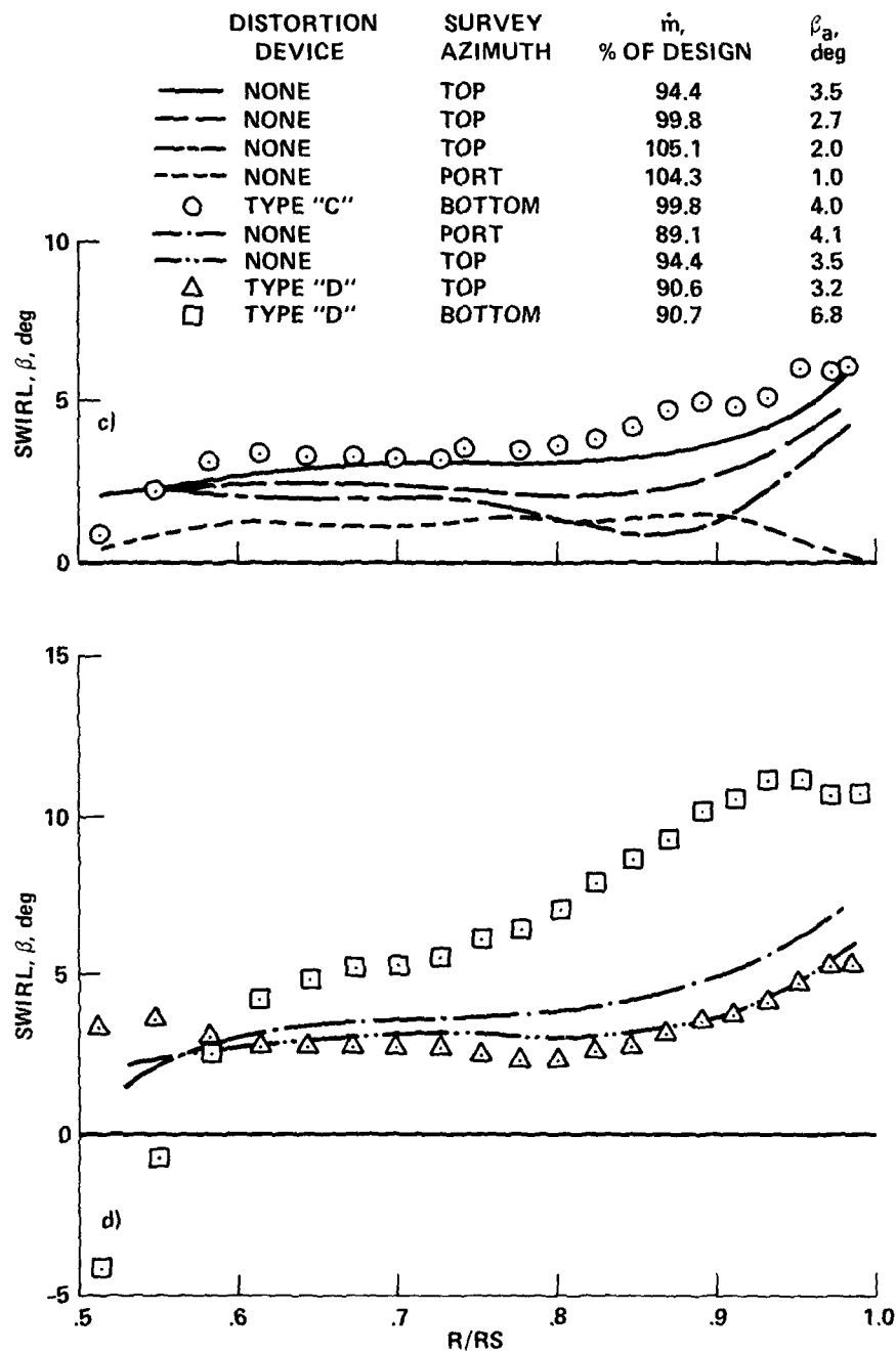
(c) Type C distortion. (d) Type D distortion.
