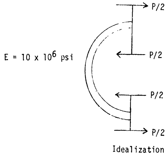
FIGURE A-12. DAMPER LUG
