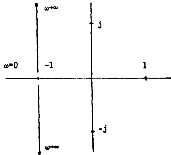
Fig. 5 Example 1 z-plot
