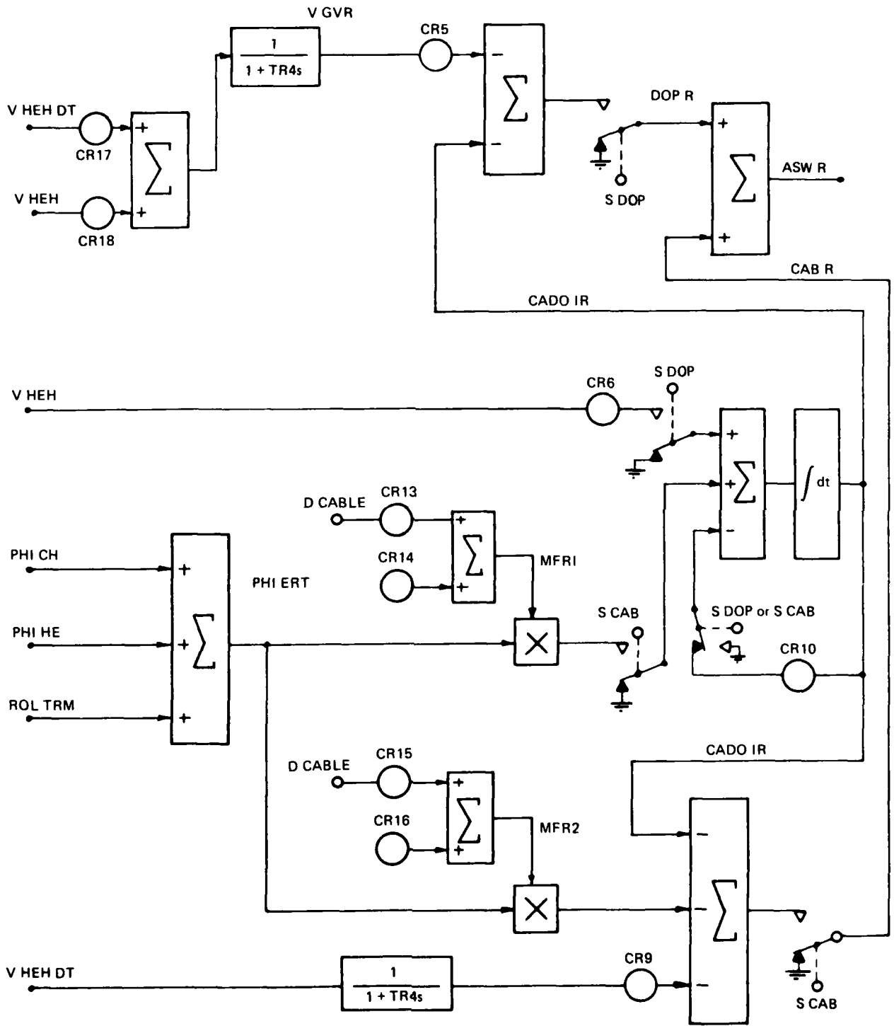
FIG 12. AFCS ASW MODE (ROLL CHANNEL)
