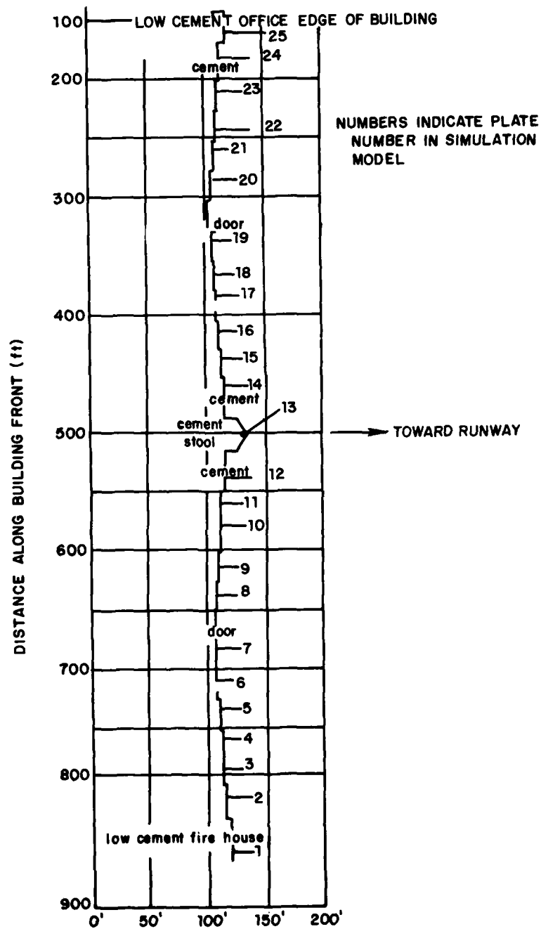
Fig. 3-114. Bldg 206 profile.
