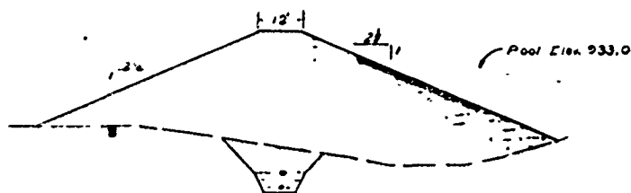
STA. 0+50 E
