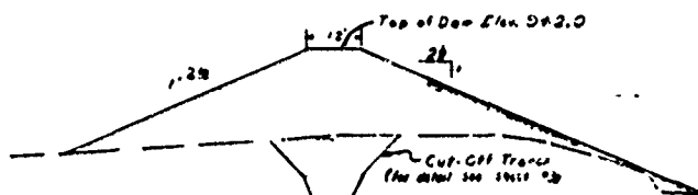
STA. 0+00
