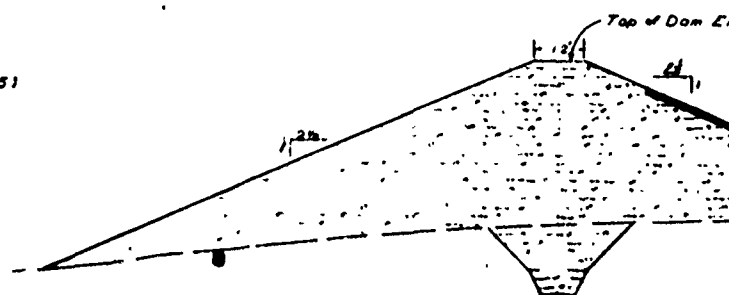
STA. 1+50 E
