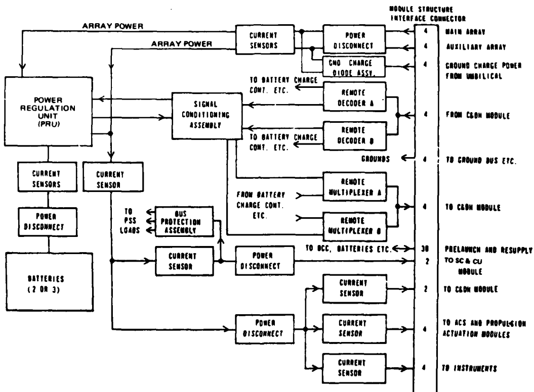
Fig. B-3—MMS block diagram--power subsystem module
