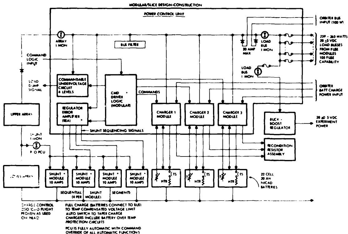
Fig. B-2 — STPSS power subsystem
