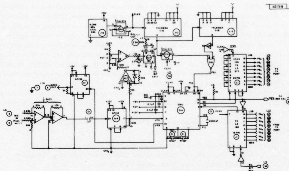
Fig. 11. PCM subsystem.
