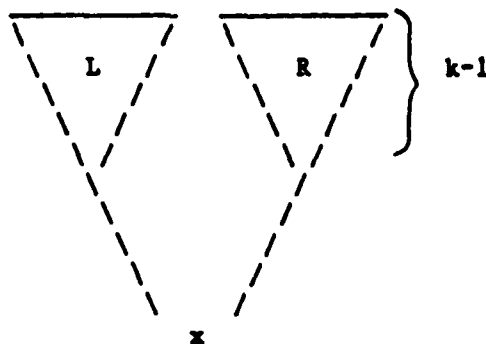
Figure 4.3 The 2SSG S.
