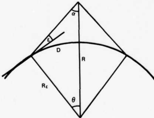
Fig. 2 — Antenna parameters
