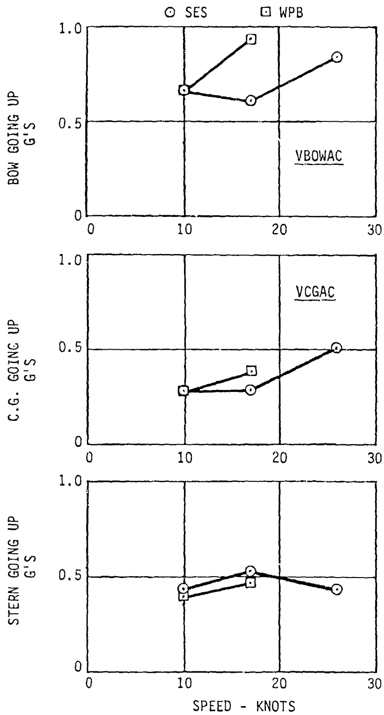
(d) Vertical Acceleration in Sea State 4 (Avg. 1/3 Highest)
