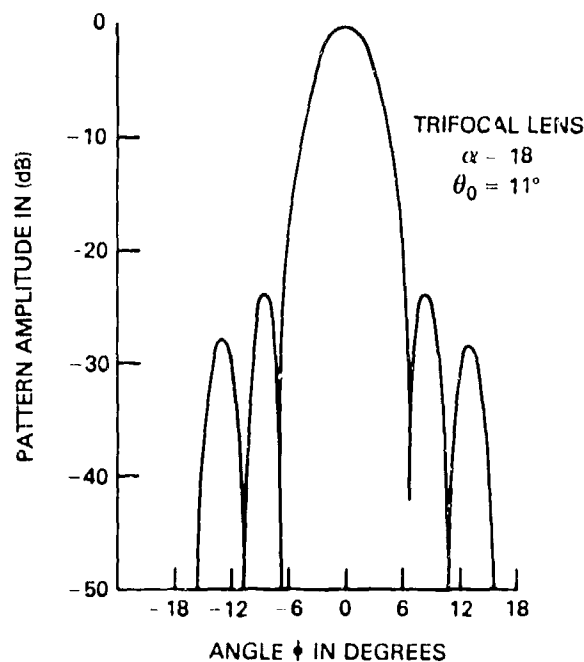
Fig. 19 — \phi -plane pattern
