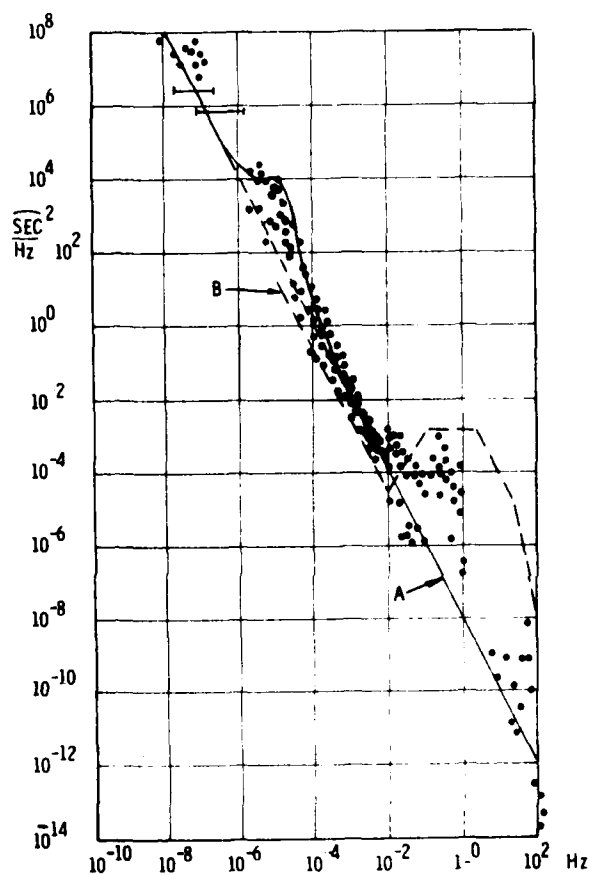
FIG. 5 COMPOSITE SPECTRUM
