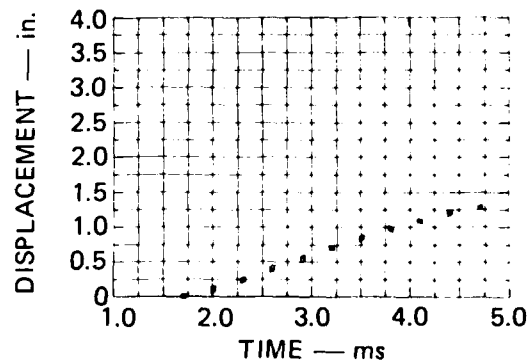
(d) SPRINGLINE DISPLACEMENT AT REFLECTING WALL TEST 17
