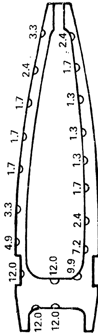
LONGITUDINAL CRACKS
