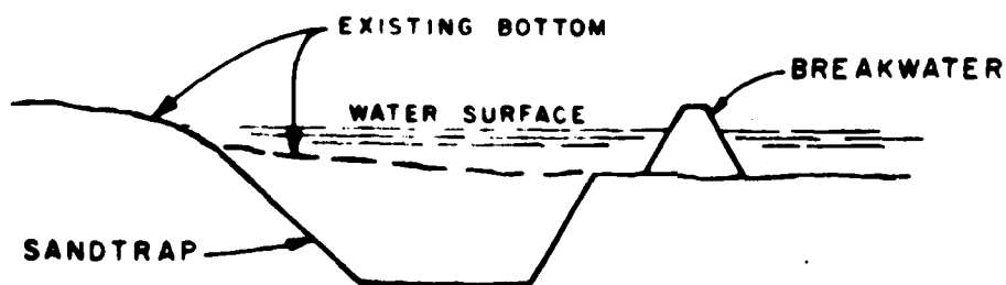
SANDTRAP SECTION (N.T.S.)
